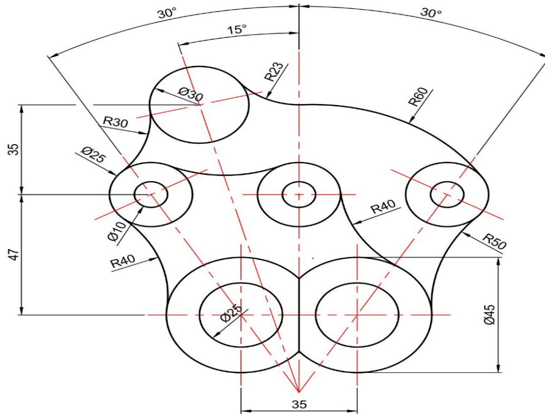
DEKPLAAT SKAAL 1:1
